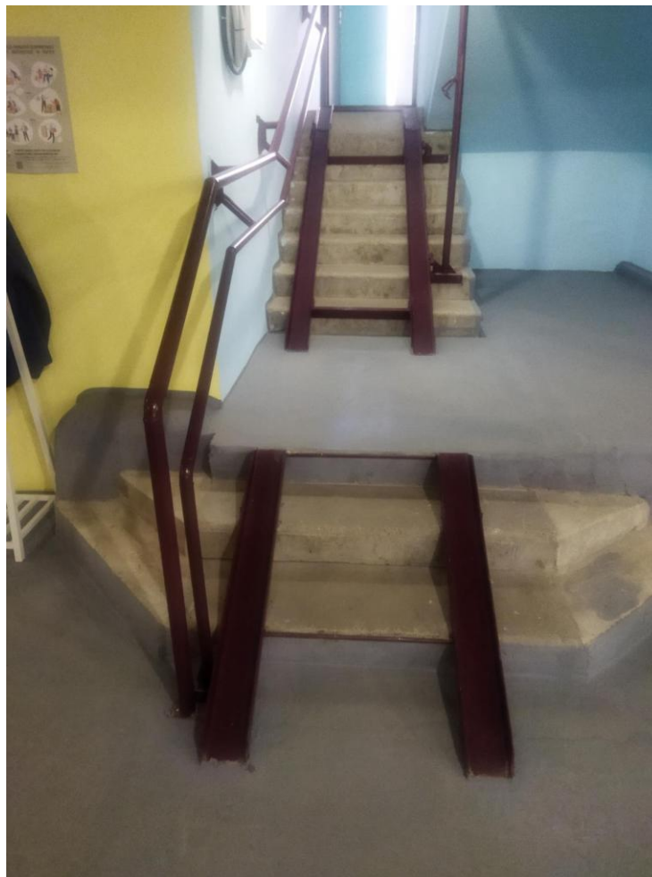
Встановлення елементів доступності СЦЗ подвійного призначення в будівлі Слов'янського ЗЗСО I-III ступенів № 15
