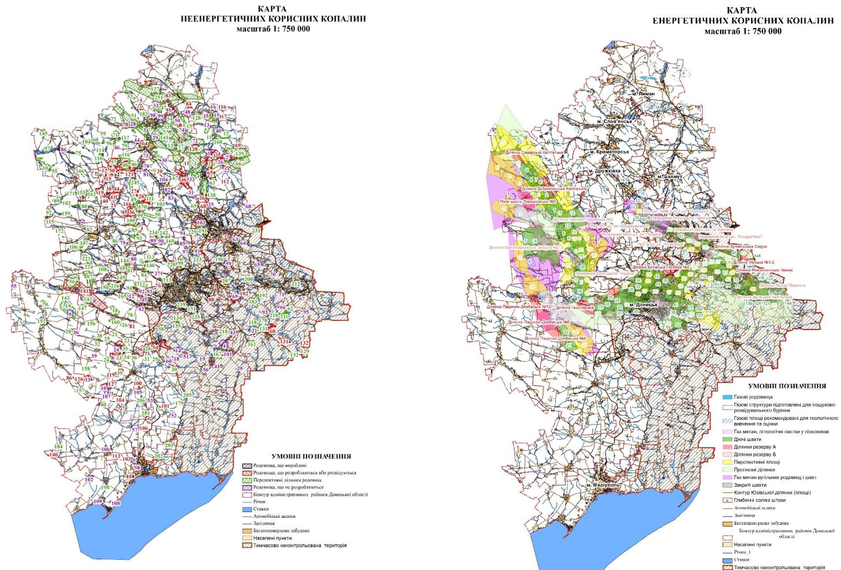
Рис. 1.6. Мапи корисних копалин Донецької області
